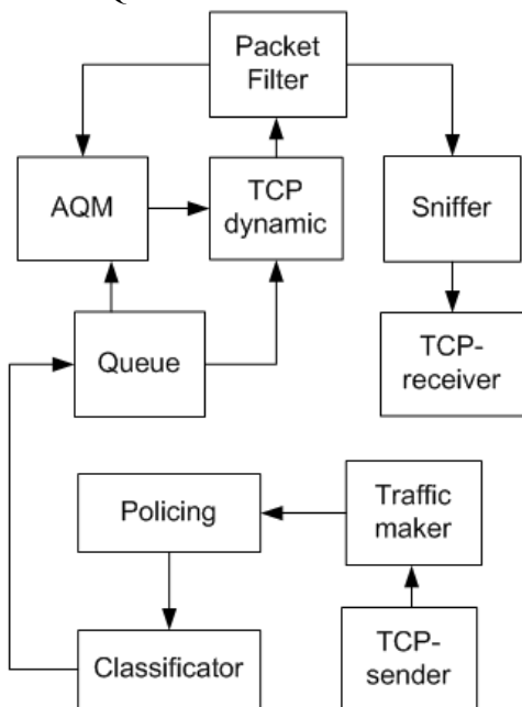
Рисунок 4 – Структурна схема експериментальної мережі
