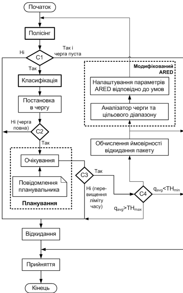
Рисунок 3 – Схема прийняття пакету на обслуговування із застосуванням модифікованого ARED
