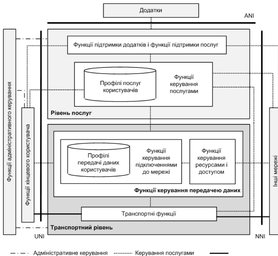
Рисунок 1 – Узагальнена функціональна архітектура NGN (ITU-T Y.2012)
