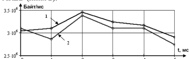
Рисунок 5 – Швидкість передачі даних r(t)
