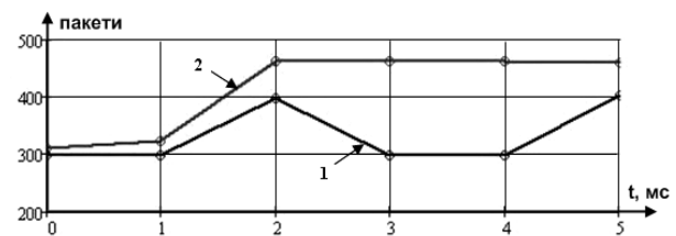
Рисунок 6 – Максимальна довжина буферної черги маршрутизатора q(t)
