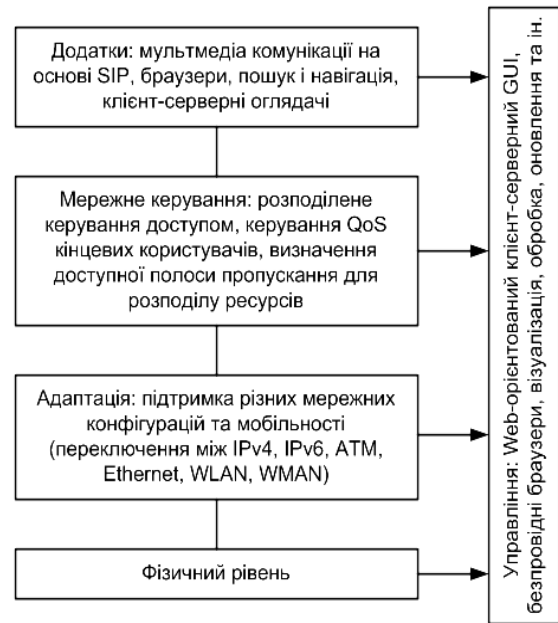
Рисунок 2 – Схема функцій QoS у мережах NGN
