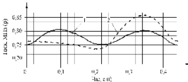
Рисунок 6 – Діаграми зміни тиску у нагнітальному патрубку розчинонасоса: 1 – диференціальний режим роботи; 2 – режим одинарної дії
