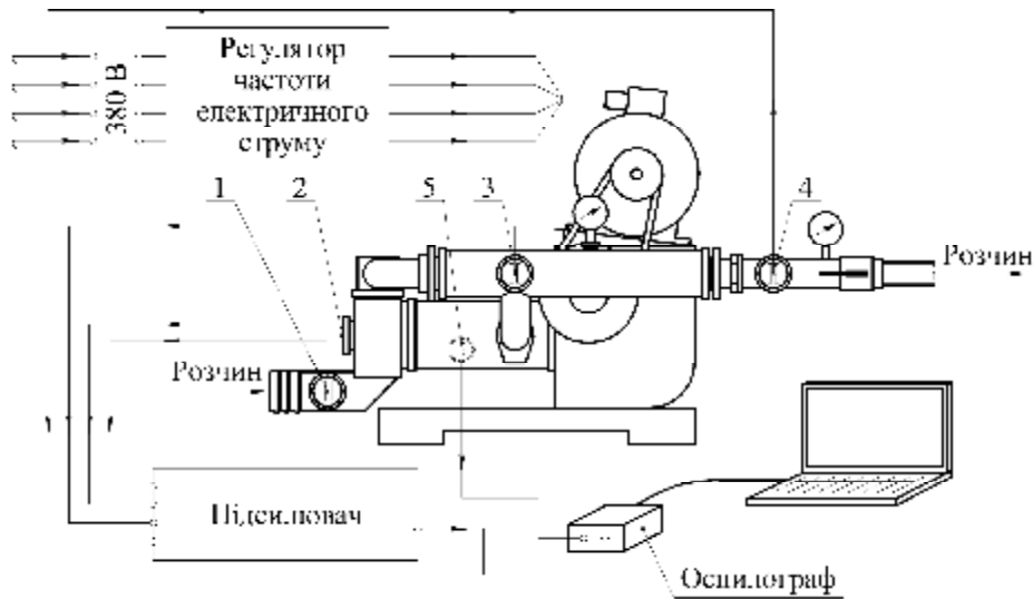
Рисунок 1 – Схема встановлення вимірювального обладнання: 1, 2, 3, 4 – місця встановлення тензOMETричних датчиків тиску, відповідно 1 – усмоктувальний патрубок; 2 – усмоктувальна робоча камера; 3 – робоча камера компенсатора; 4 – нагнітальний патрубок; 5 – датчик переміщення
