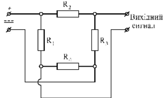
Рисунок 3 – Мостова схема підключення тензометричних датчиків
