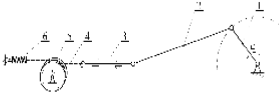
Рисунок 4 – Схема встановлення датчика переміщення: 1 – кривошип; 2 – шатун; 3 – допоміжний стрижень; 4 – капронова струна; 5 – регульований резистор із встановленим на його осі шківом; 6 – пружина розтягування
