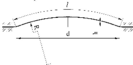
Рисунок 2 – Схема вимірювання вихідних даних для розрахунку величини відносної деформації e , % діафрагми
