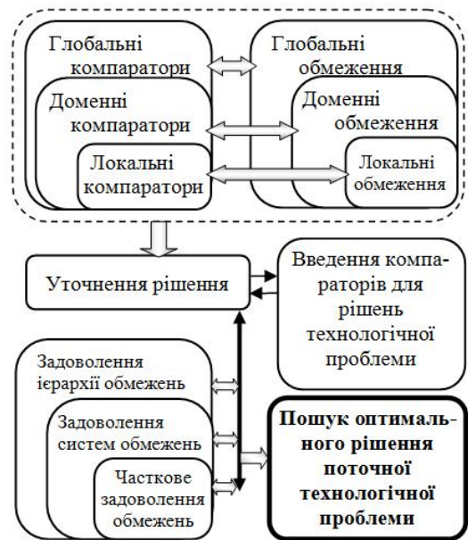
Рисунок 2 – Процедура пошуку оптимального рішення шляхом задоволення обмежень
