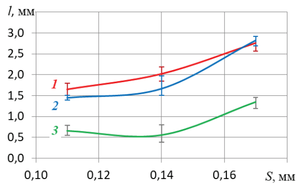
Рис. 5. Залежність довжини незрізаних волокон від величини зазору між інструментом і втулкою: а) на вході в заготовку; б) на виході з заготовки; 1- органопластик; 2 – склопластик; 3 – армований вуглепластик
