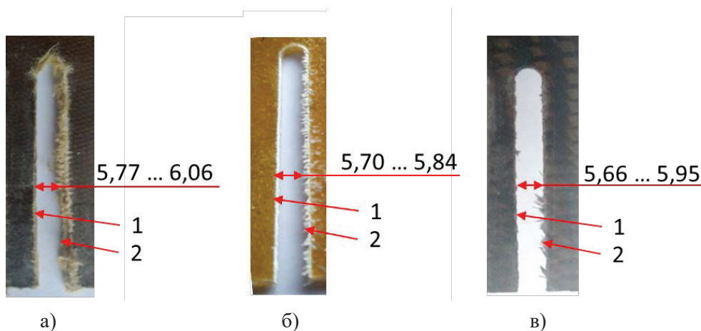
Рисунок 3 – Вимірювання ширини прорізаного паза: а) органопластик; б) склопластик; в) армований вуглепластик; 1 – вхід різального інструмента; 2 – вихід різального інструмента
