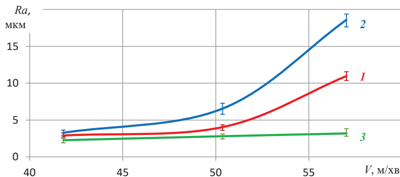
Рисунок 4 – Залежність шорсткості поверхні від швидкості різання: 1- органопластик; 2 - склопластик; 3 – армований вуглепластик
