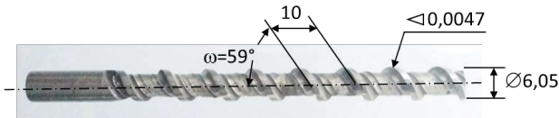
Рисунок 2 – Різальний інструмент з гвинтовим зубом
