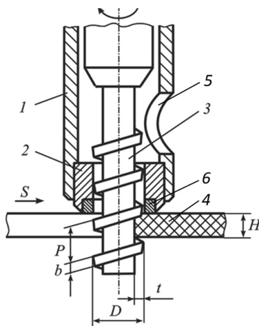
Рисунок 1 – Схема пристрою для обрізання листових композитів
